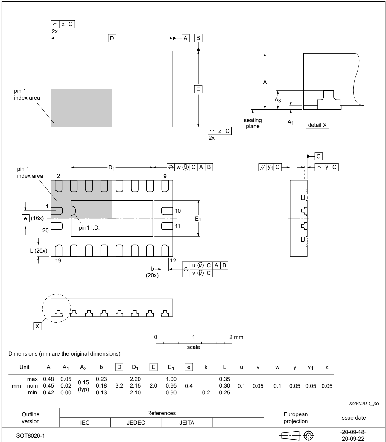
Fig. 1. Package outline DHXQFN (SOT8020-1)
