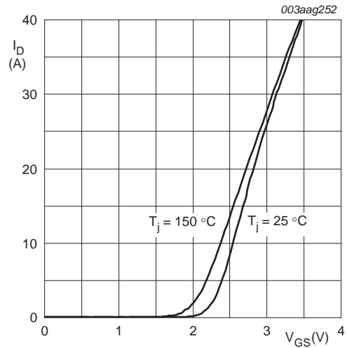
V_{DS} = 10V
