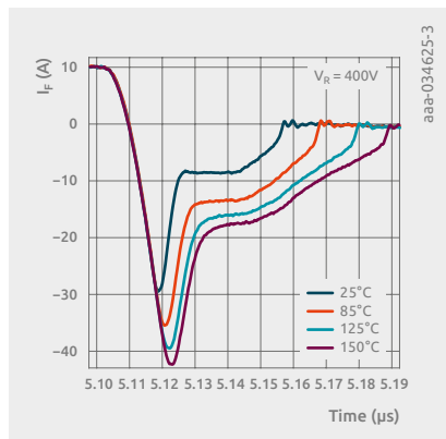
Si diode
